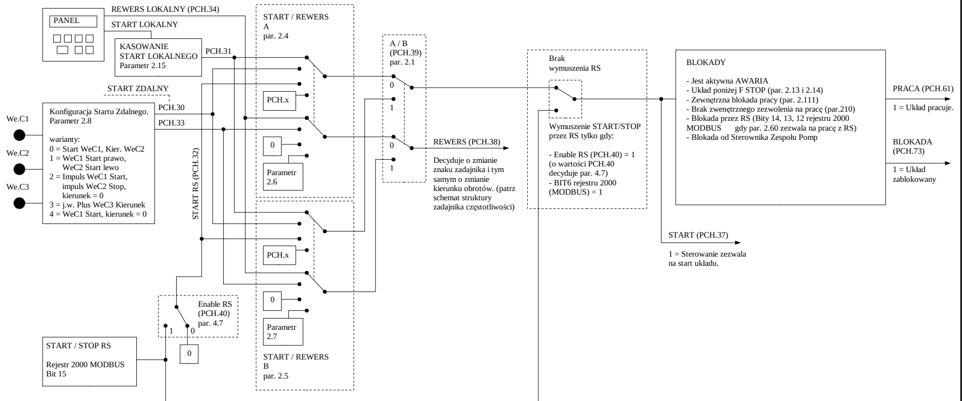
Rys. 4.2c - Pełna struktura sterowania MFC710/AcR Sekcja sygnału START / STOP, blokady pracy i sterowania kierunkiem obrotów
