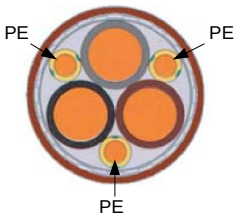
Rys. 2.2 Przekrój kabla HELUKABEL TOPFLEX-EMV-3 PLUS-2YSLCY-J 600/1000 V
